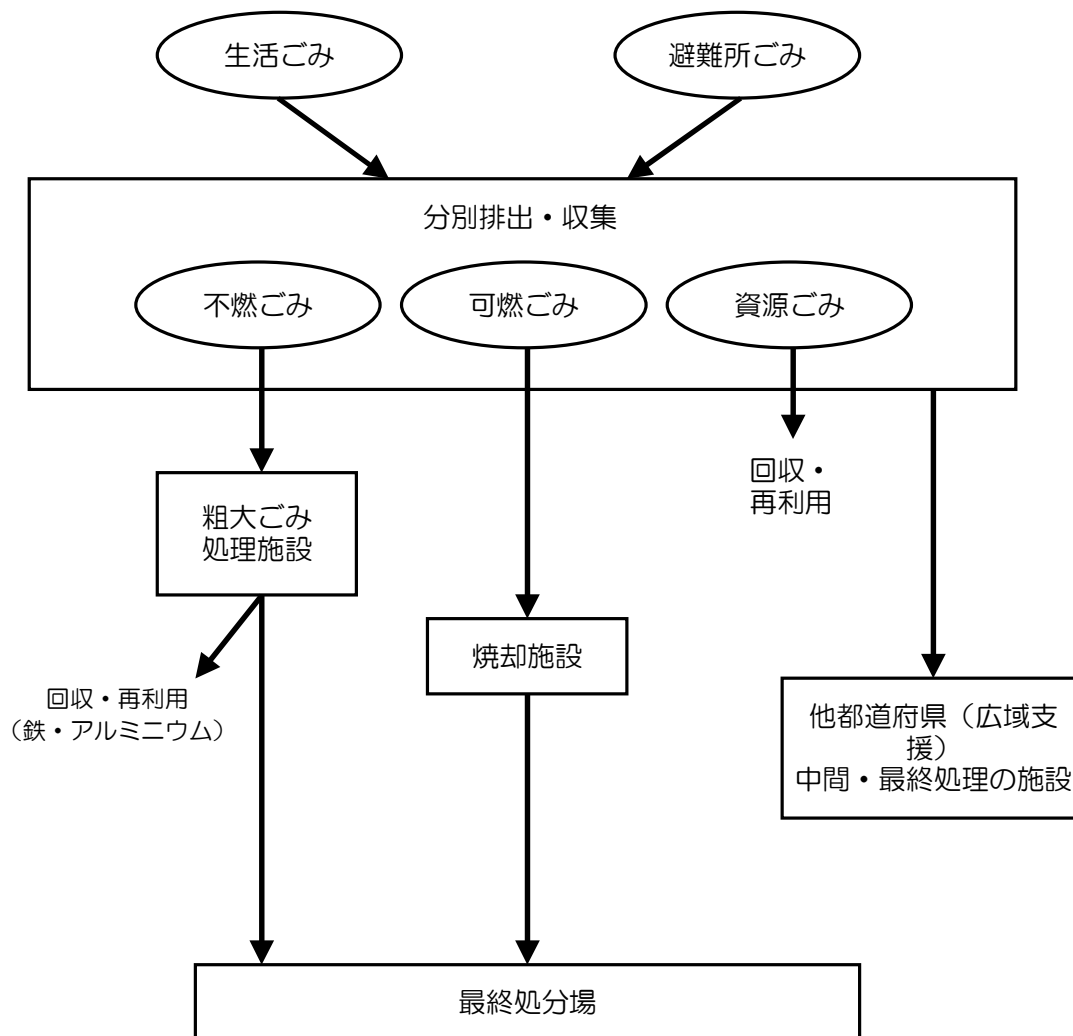
図表1－12 生活ごみ・避難所ごみの処理の流れ
