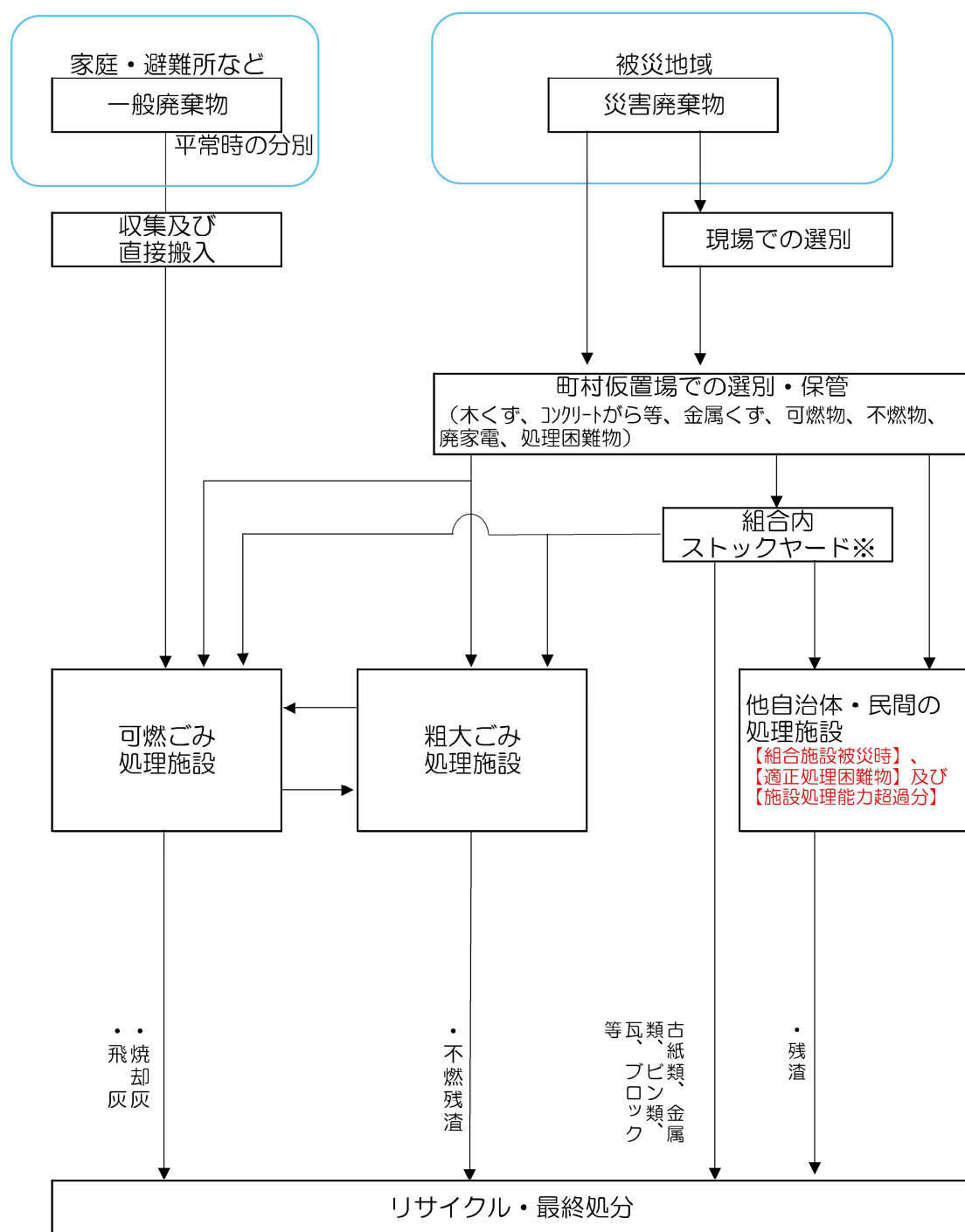
図表6－13 災害廃棄物の処理フロー
